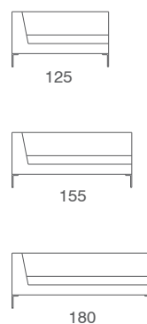
Elemento laterale dx o sx Right or left unit
